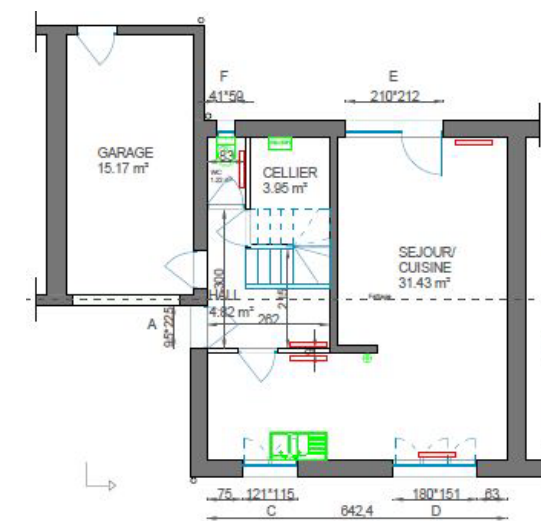
PLAN RDC - T5
